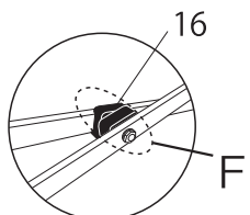
※2 拡大図
